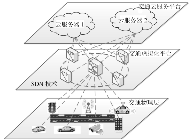
图 4 智能交通云控制网络虚拟化架构
