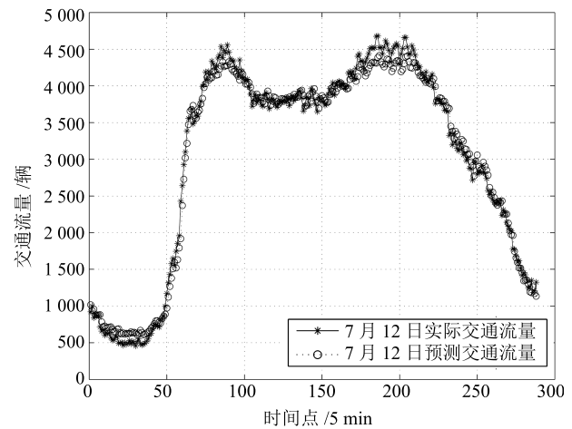
图 10 BP-BELM 预测交通流与实际交通流的对比 Fig. 10 Comparison of BP-BELM prediction traffic flow and actual traffic flow
