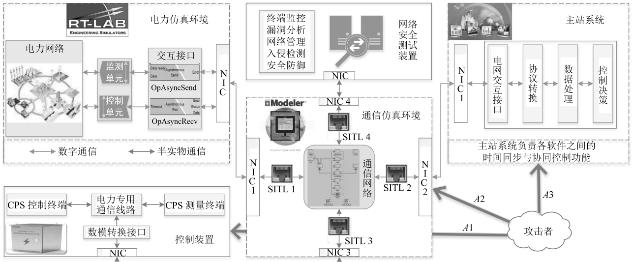
图5 电力CPS网络联合攻防平台框架
